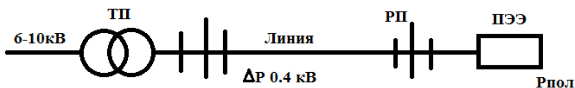
Фиг.1. Упрощенная схема электроснабжения рассредоточенных объектов
